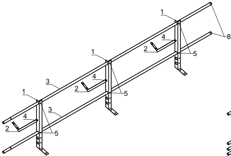
Ограждение РП-ОГ-УПР-600
