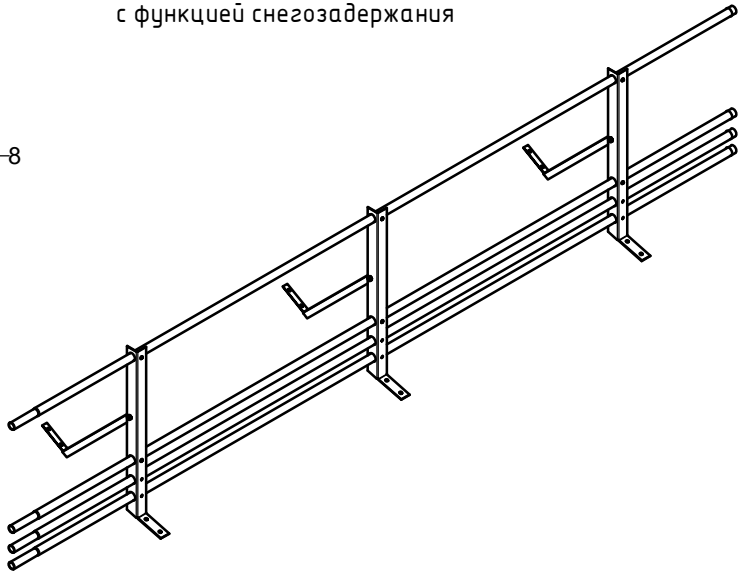
Ограждение РП-ОГ-УПР-600 с функцией снегозадержания
